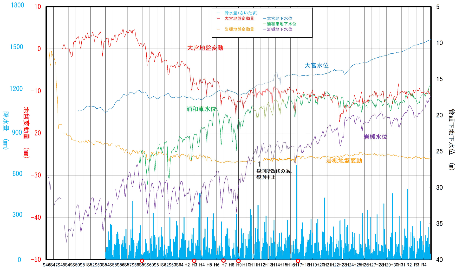
図-2.3.1 地盤沈下・地下水位 経年年化図
